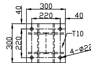
Part E Scale: 1.5: 1
