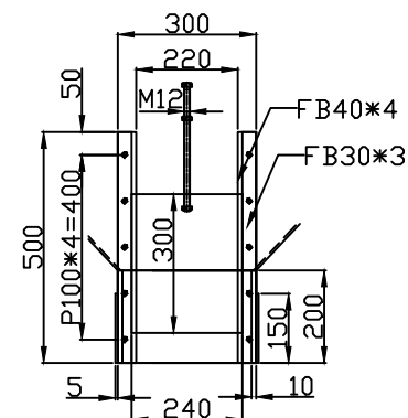
Part F Scale: 1.5: 1
